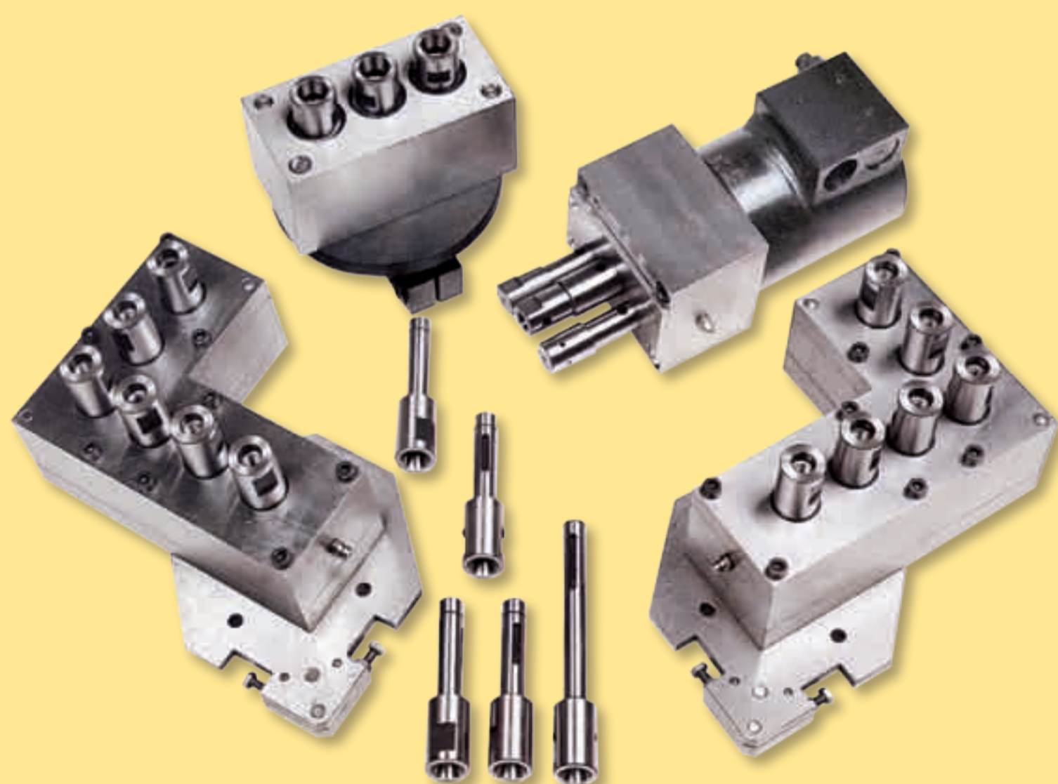
GŁOWICE WIERTARSKIE WIELOWRZECIONOWE
